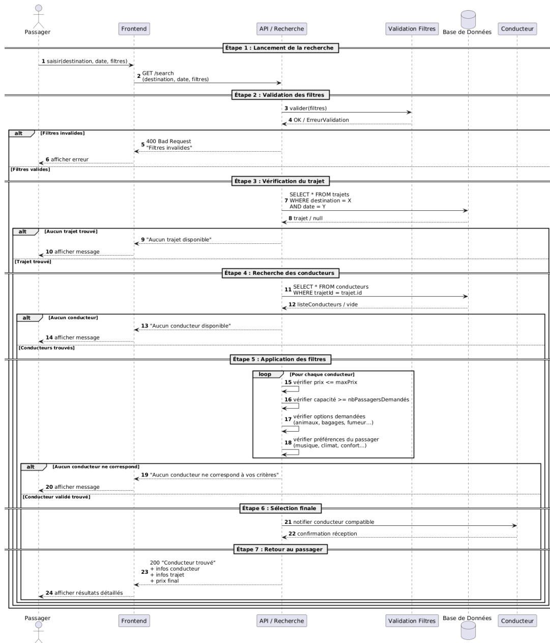
Diagramme de séquence qui décrit le déroulement des échanges entre les composants lors de la recherche d'un trajet par un utilisateur
